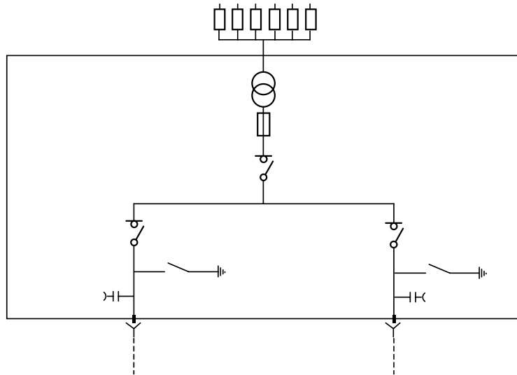
Figura 2: Esquema unifilar
